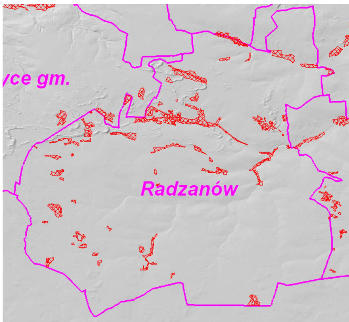
Rysunek 16. Gleby organiczne, na tle ukształtowania terenu Gminy Radzanów.
